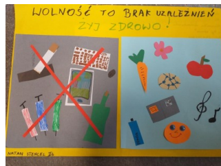
Wvroznienie Natan
